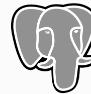
Postgre SQL
